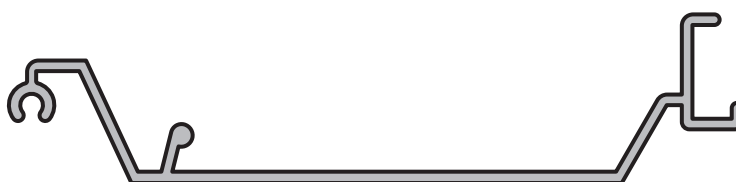
TAPACINTA Perfil: 129 Peso: 0,589 Kg/m Matriz: M1848
