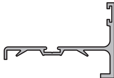
TAPACANTO CON TOPE PARA BATIENTE Perfil: 42 Peso: 0,481 Kg/m Matriz: M0799
