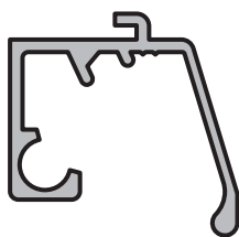
BISAGRA TAPACINTA Perfil: 128 Peso: 0,343 Kg/m Matriz: M1847
