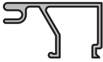
CONTRAVIDRIO Perfil: 205 Peso: 0,199 Kg/m Matriz: M2693
