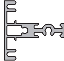
TRAVESAÑO VIDRIO REPARTIDO Perfil: M-2665 Peso: 0,562 Kg/m Matriz: M2665
