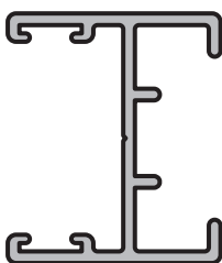
CIERRE CENTRAL - PUERTA Y VENTANA
