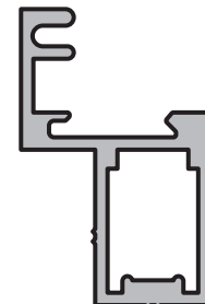
HOJA SECUNDARIA PUERTA Perfil: 136 Peso: 0,497 Kg/m Matriz: M1876
