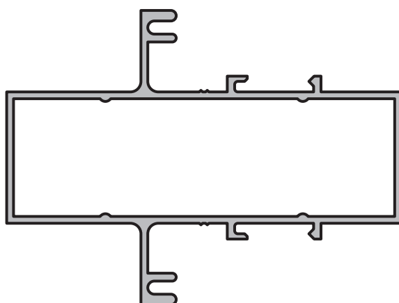
TRAVESAÑO - PAÑO FIJO Perfil: 94 Peso: 0,975 Kg/m Matriz: M1366
