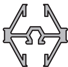
TRAVESAÑO VIDRIO REPARTIDO Perfil: 801 Peso: 0,434 Kg/m Matriz: M2775
