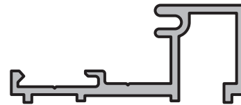
PORTA CONTRAVIDRIOS Perfil: 43 Peso: 0,429 Kg/m Matriz: M0844
