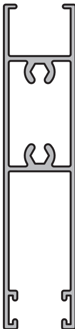
TRAVESAÑO HOJA PUERTA CORREDIZA Perfil: 224 Peso: 0,915 Kg/m Matriz: M2741
