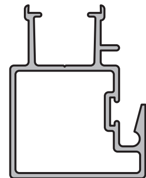
PARANTE CENTRAL REFORZADO HOJA Perfil: 54 Peso: 0,729 Kg/m Matriz: M0949
