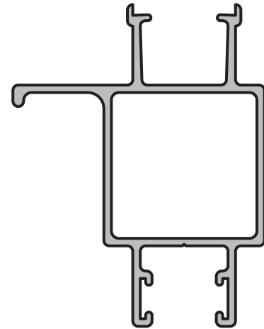
PARANTE LATERAL REFORZADO - PUERTA CORREDIZA Perfil: 220 Peso: 0,821 Kg/m Matriz: M2673
