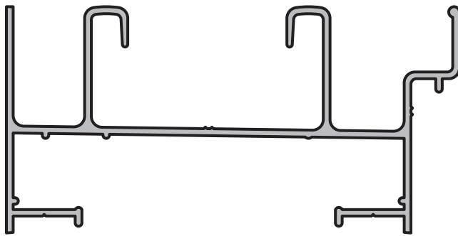
MARCO - VENTANA Y PUERTA CORREDIZA
