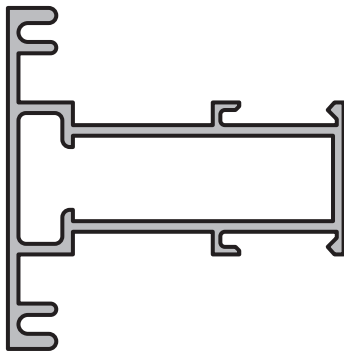
TRAVESAÑO PARA VIDRIO PARTIDO Perfil: 209 Peso: 0,718 Kg/m Matriz: M2697
