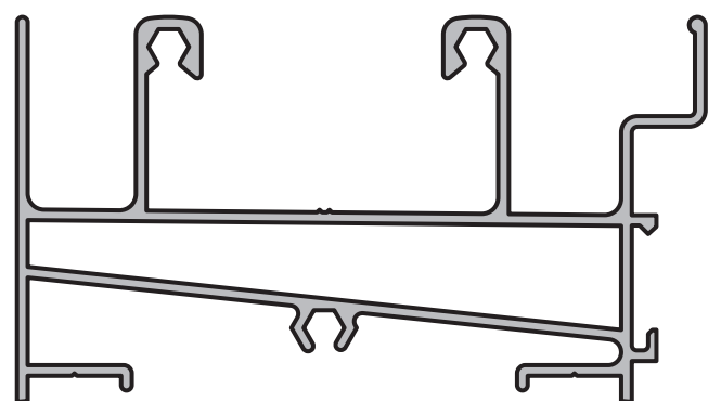
UMBRAL CON CAJA DE AGUA CORREDIZA
